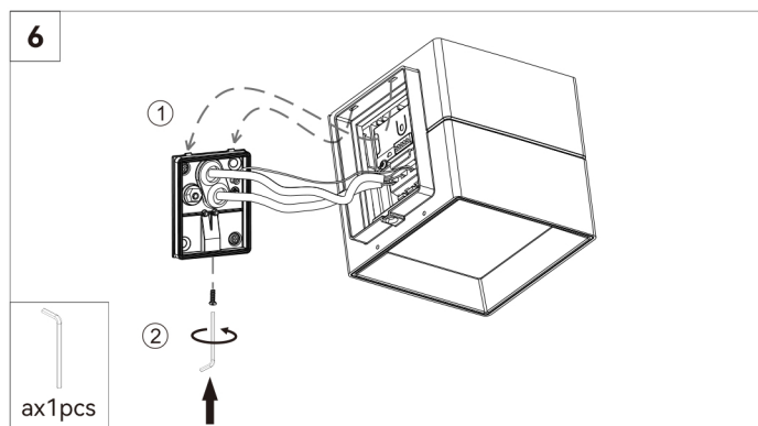
Lampengehäuse auf die Montageplatte legen und von unten mit Schraube befestigen.
