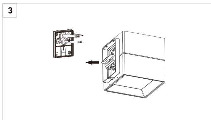
Terminalschublade ausfahren.
