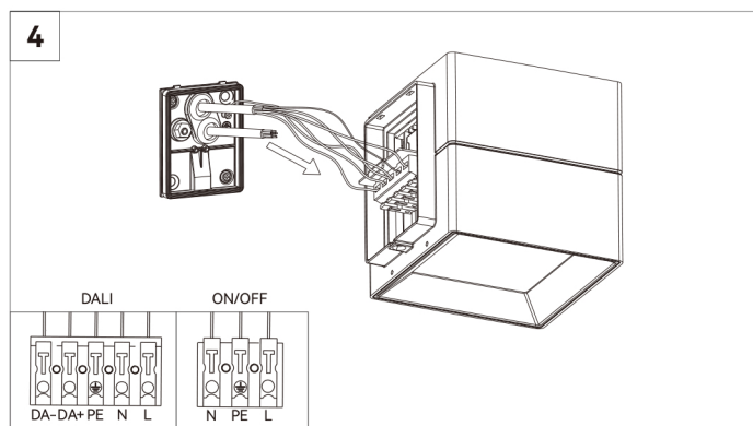
Stromlos schalten, Anschlusskabel verbinden.
