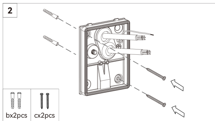
Führen sie das Anschlusskabel durch die Montageplatte und montieren sie die Platte an der Wand.
