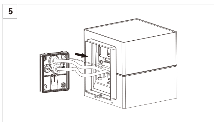
Nach Anschluss - Terminalschublade in Lampengehäuse schieben.
